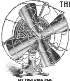
500 VOLT DESK FAN.
