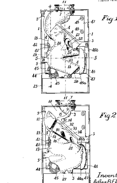
A. B. FLAGG & W. H. LIVERMORE ONE SLOT PAY STATION PATENTED APR. 22, 1912
