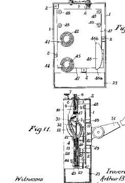
A. B. FLAGG & W. H. LIVERMORE ONE SLOT PAY STATION PATENTED APR. 22, 1912
